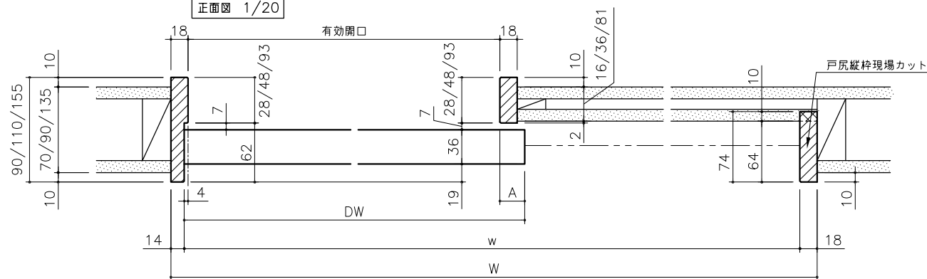
横断面図 1/4
