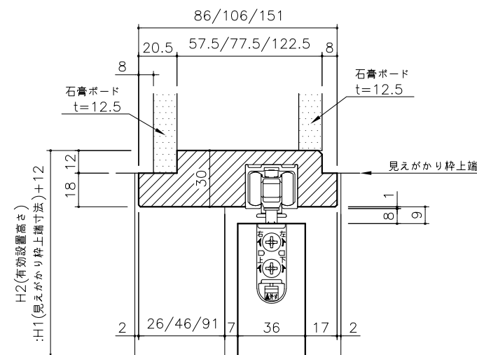
縦上部納まり詳細図 1/2
