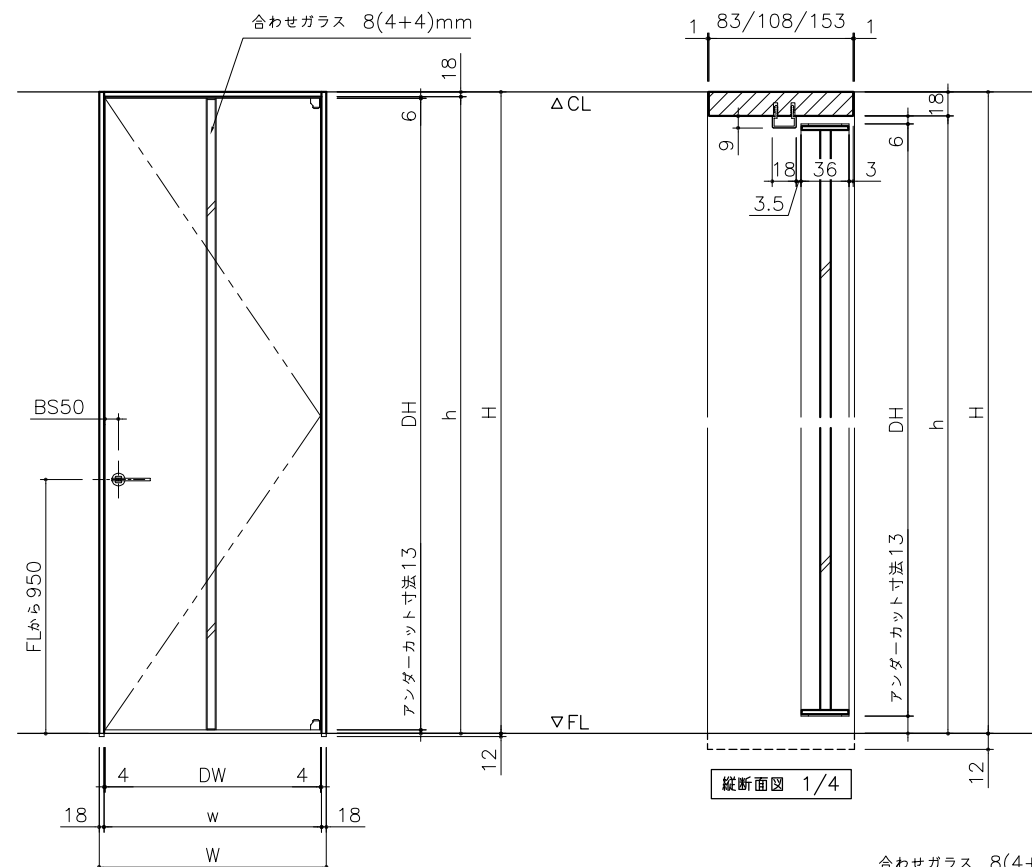
正面図 1/20
