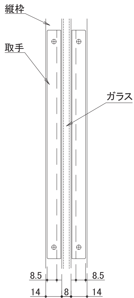
側面図
