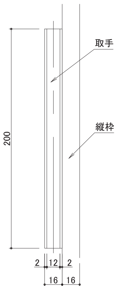
正面図
