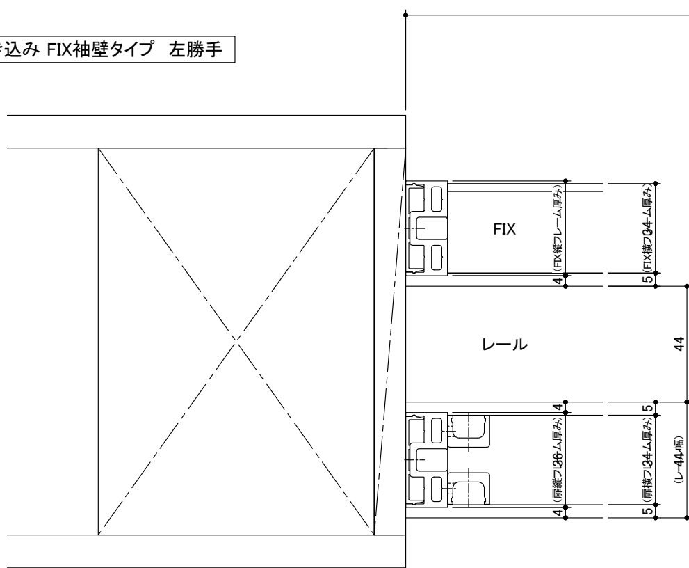
戸尻部 詳細図
