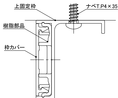
ブロンズフレーム FIX上工程枠 詳細図
