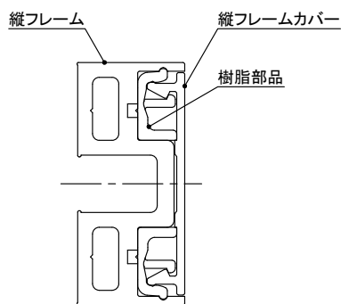
ブロンズ縦フレーム 詳細図
