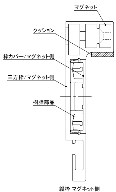
ブロンズフレーム 3方枠 詳細図
