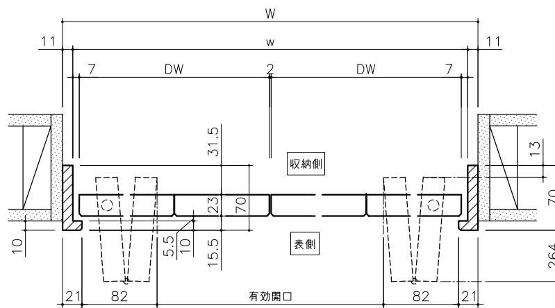
横断面図 1/4
