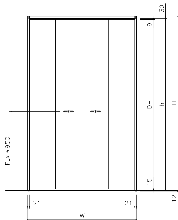
正面図 1/20
