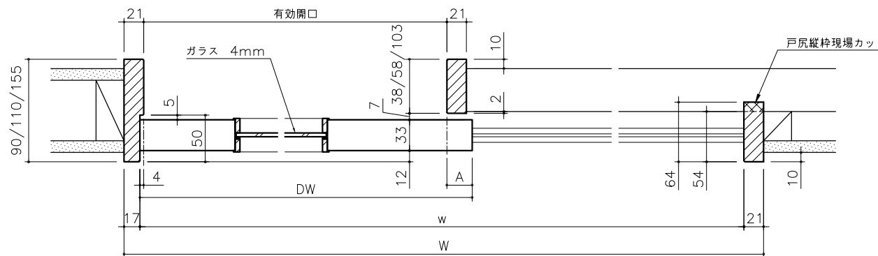
横断面図 1/4
