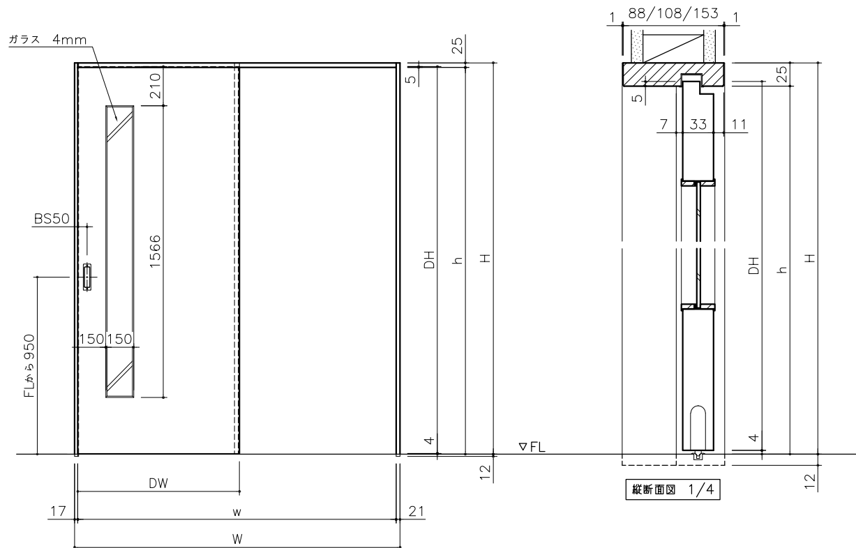
正面図 1/20
