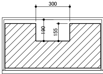
下引出し 切り欠き寸法
