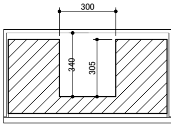
上引出し 切り欠き寸法
