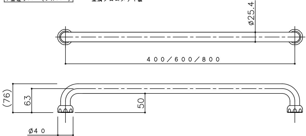
Ⅰ型握りバー（シルバー）
