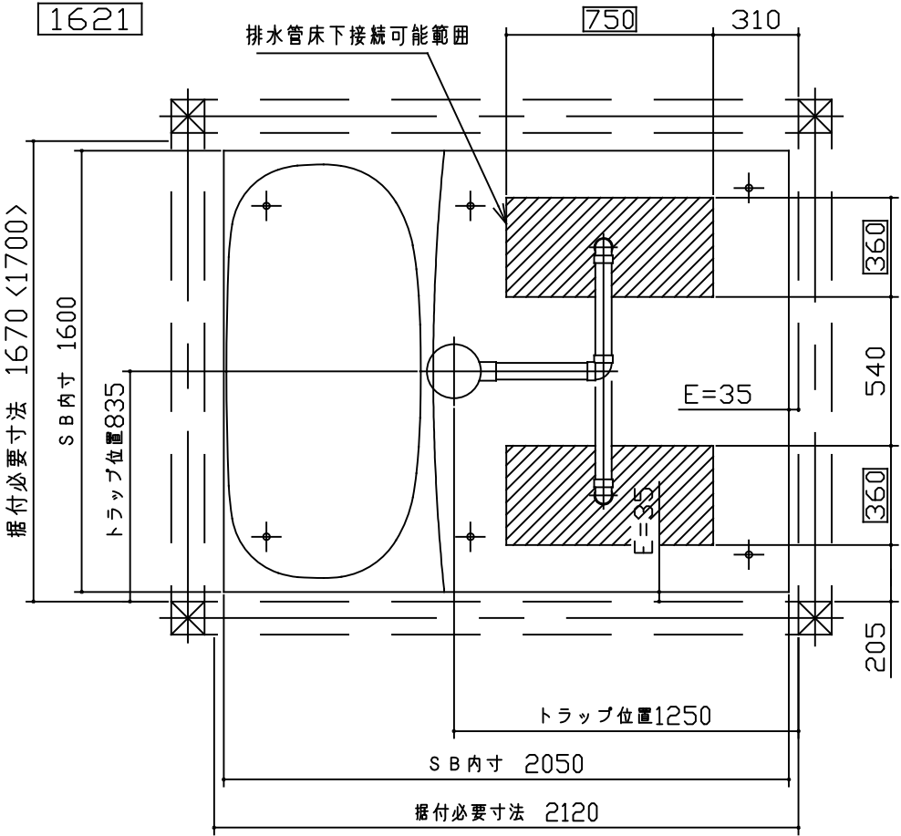
■【排水位置図】排水管落とし可能位置図（1/25）
