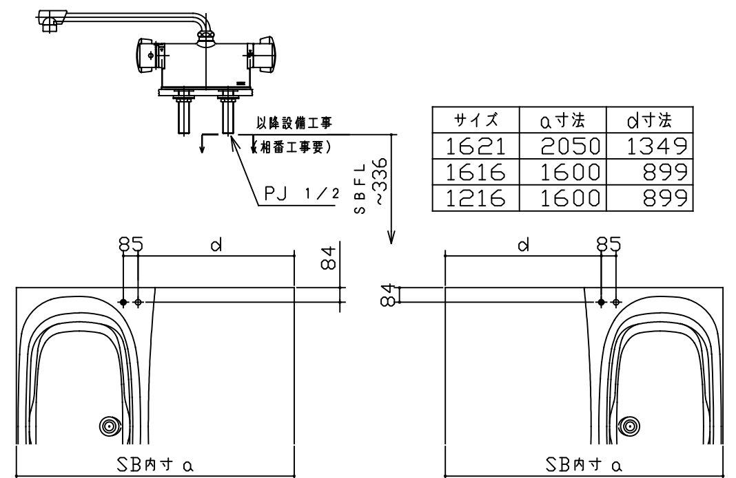
＜参考＞兼用デッキ水栓位置図
