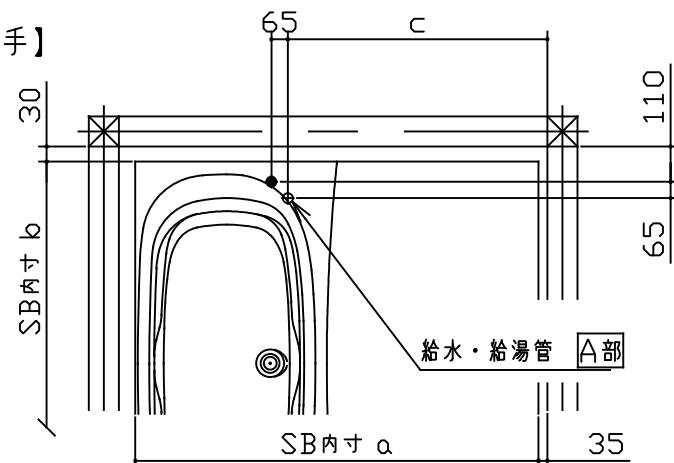
事前立ち上げ配管位置
