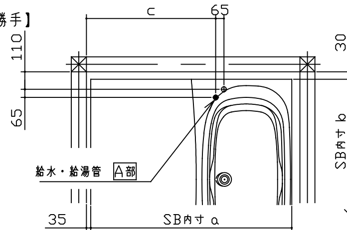
＜参考＞浴槽側デッキ水栓位置図
