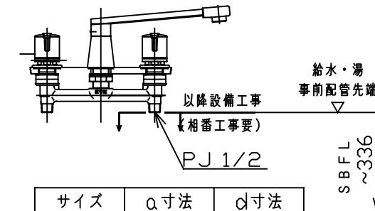
＜参考＞浴槽側デッキ水栓位置図
