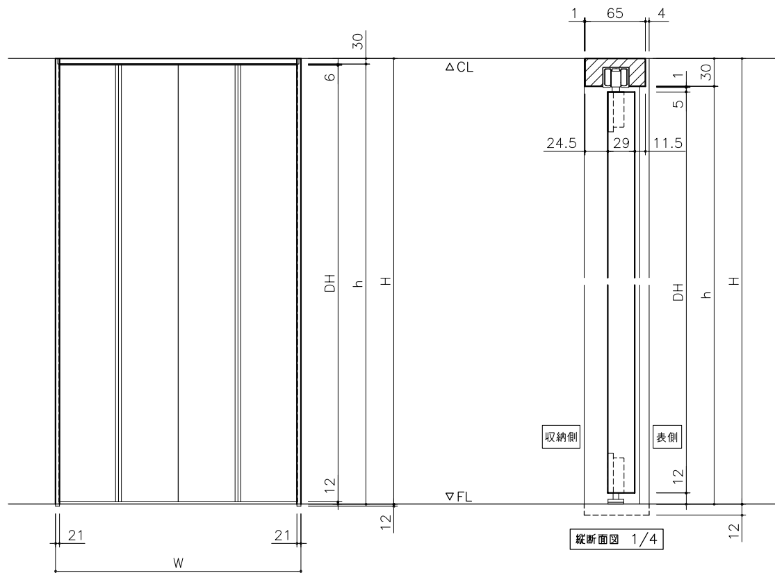
正面図 1/20
