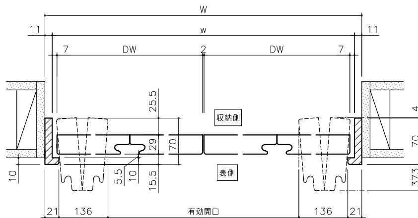
横断面図 1/4
