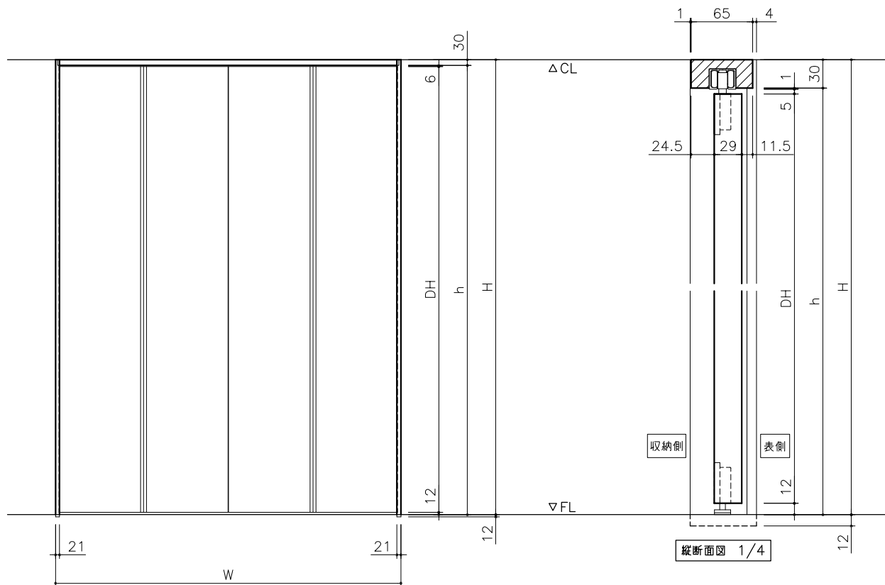
正面図 1/20
