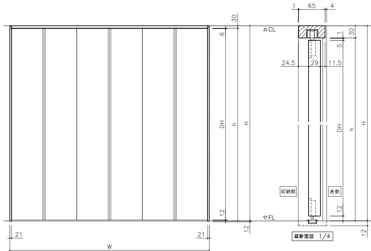
正面図 1/20
