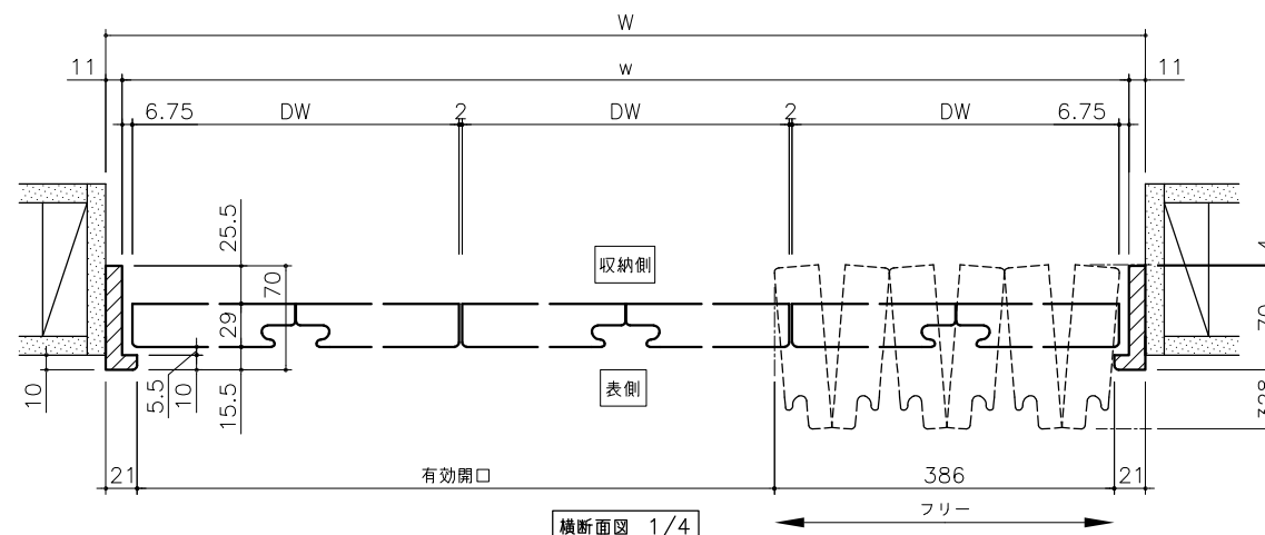
横断面図 1/4
