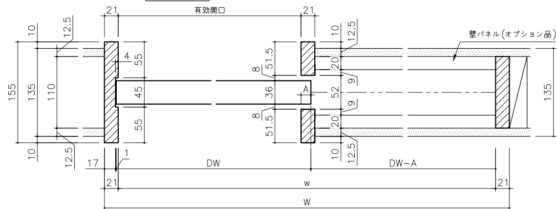
横断面図 1/4
