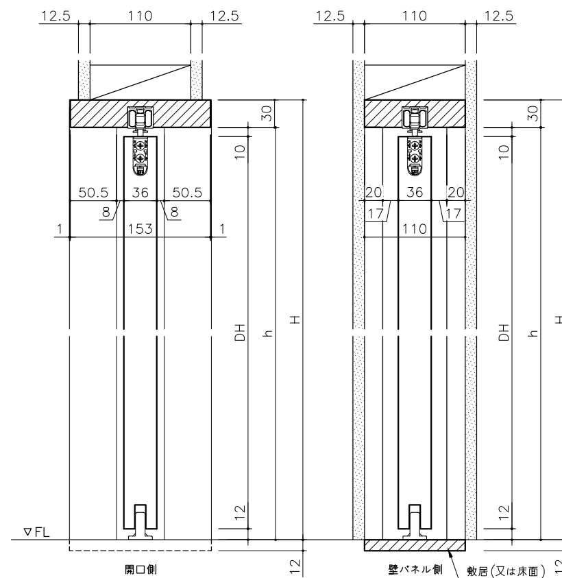
縦断面図 1/4
