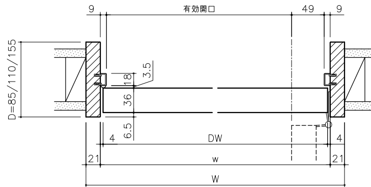
横断面図 1/4
