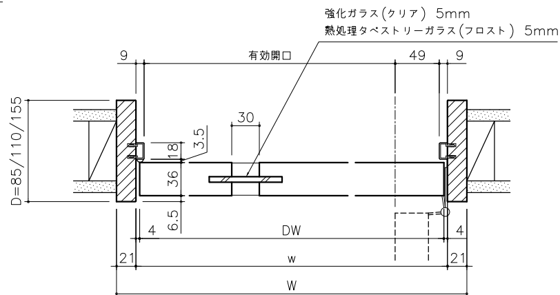
横断面図 1/4
