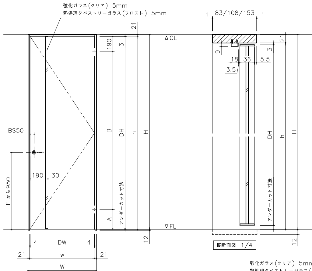
正面図 1/20
