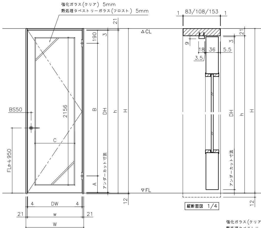
正面図 1/20
