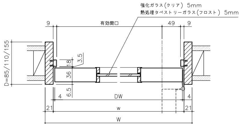
横断面図 1/4
