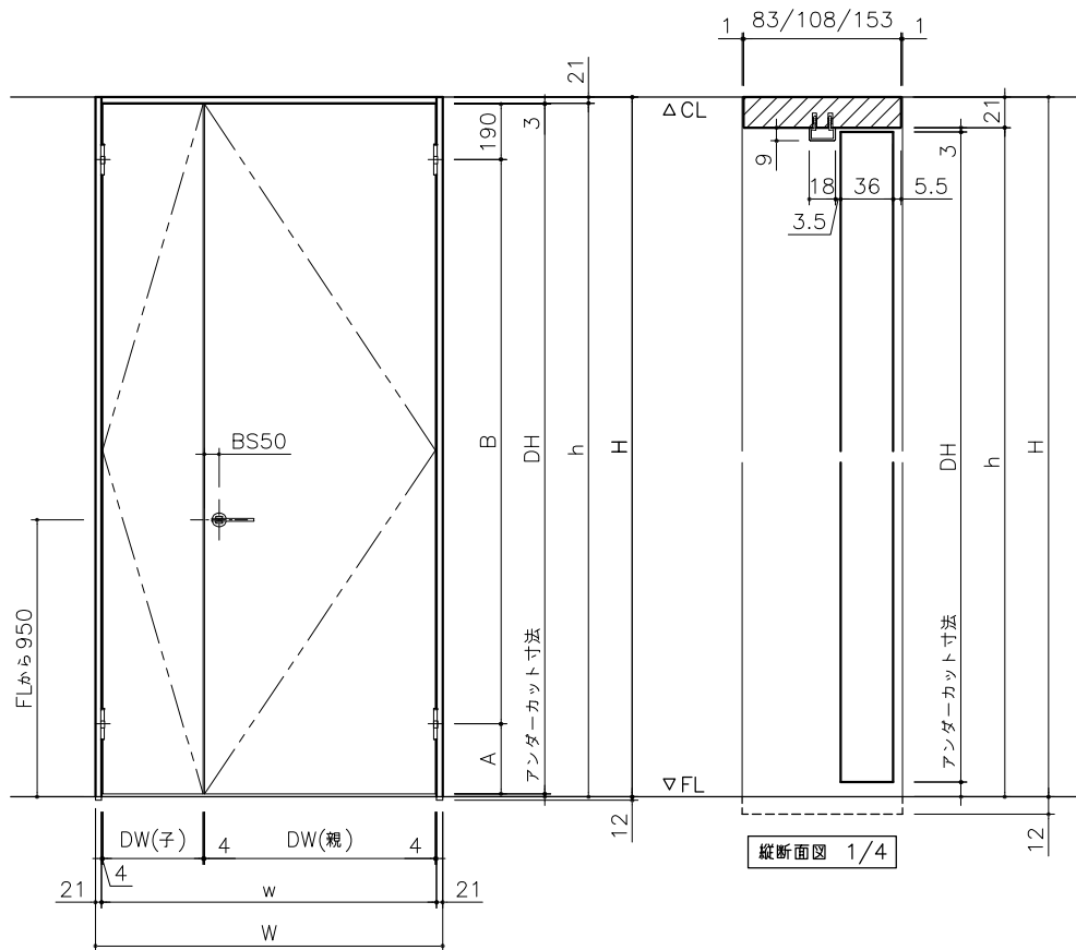
正面図 1/20
