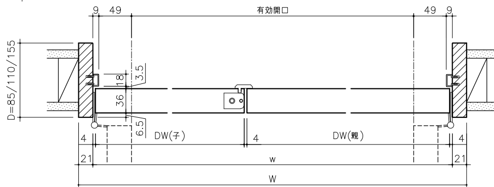
横断面図 1/4
