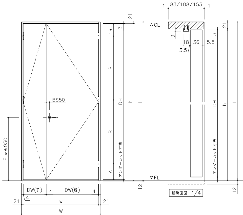
正面図 1/20
