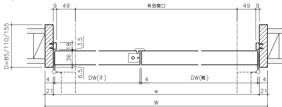
横断面図 1/4
