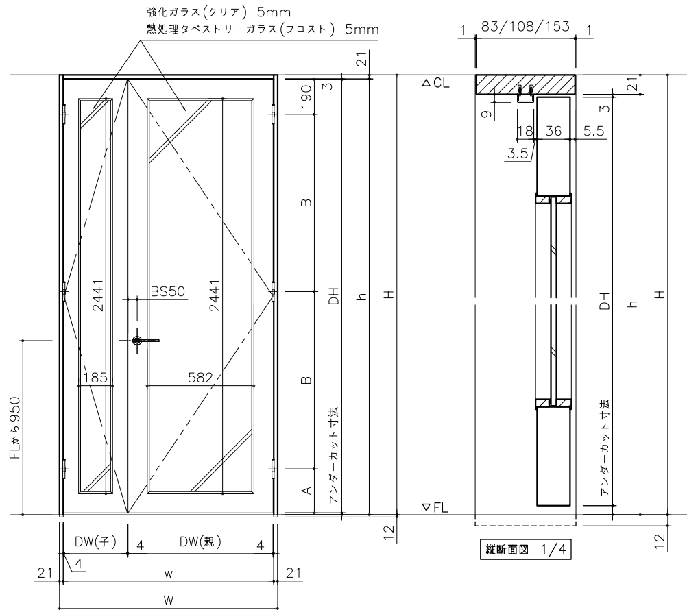
正面図 1/20
