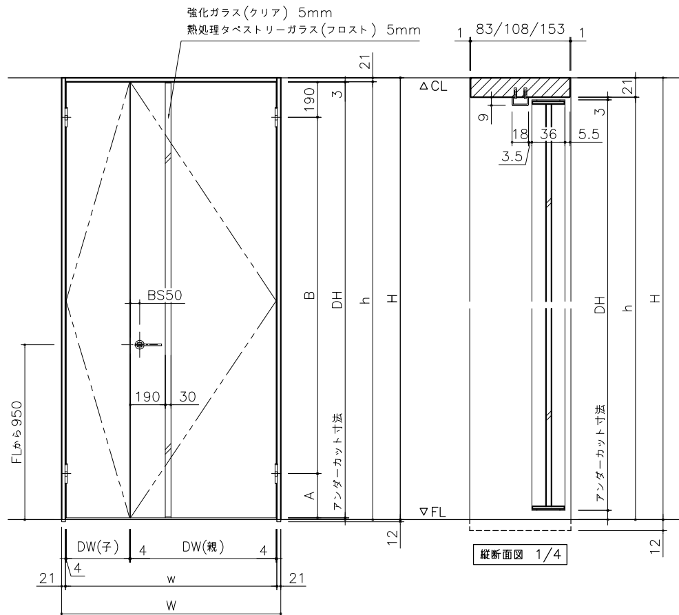
正面図 1/20
