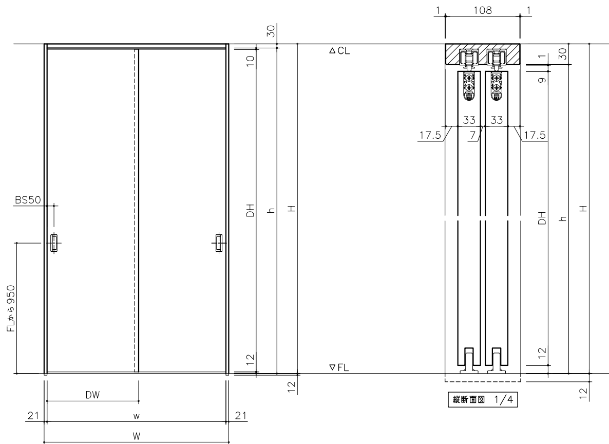
正面図 1/20
