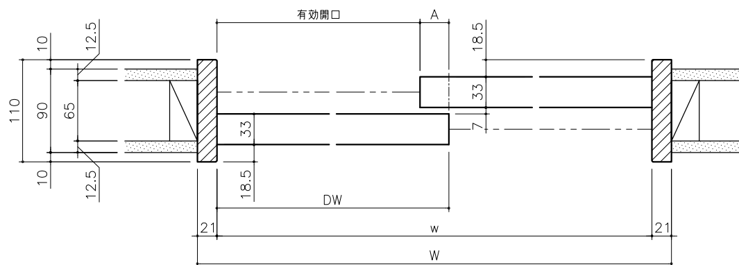
横断面図 1/4
