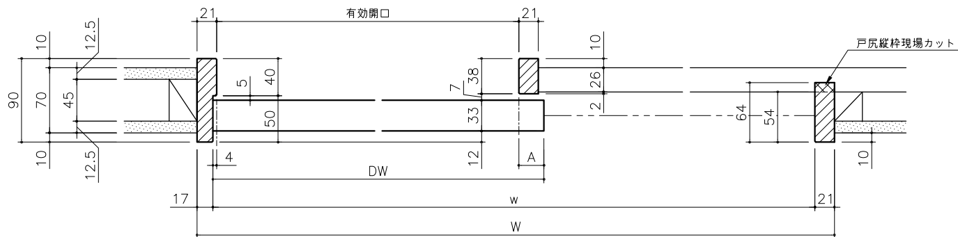
横断面図 1/4
