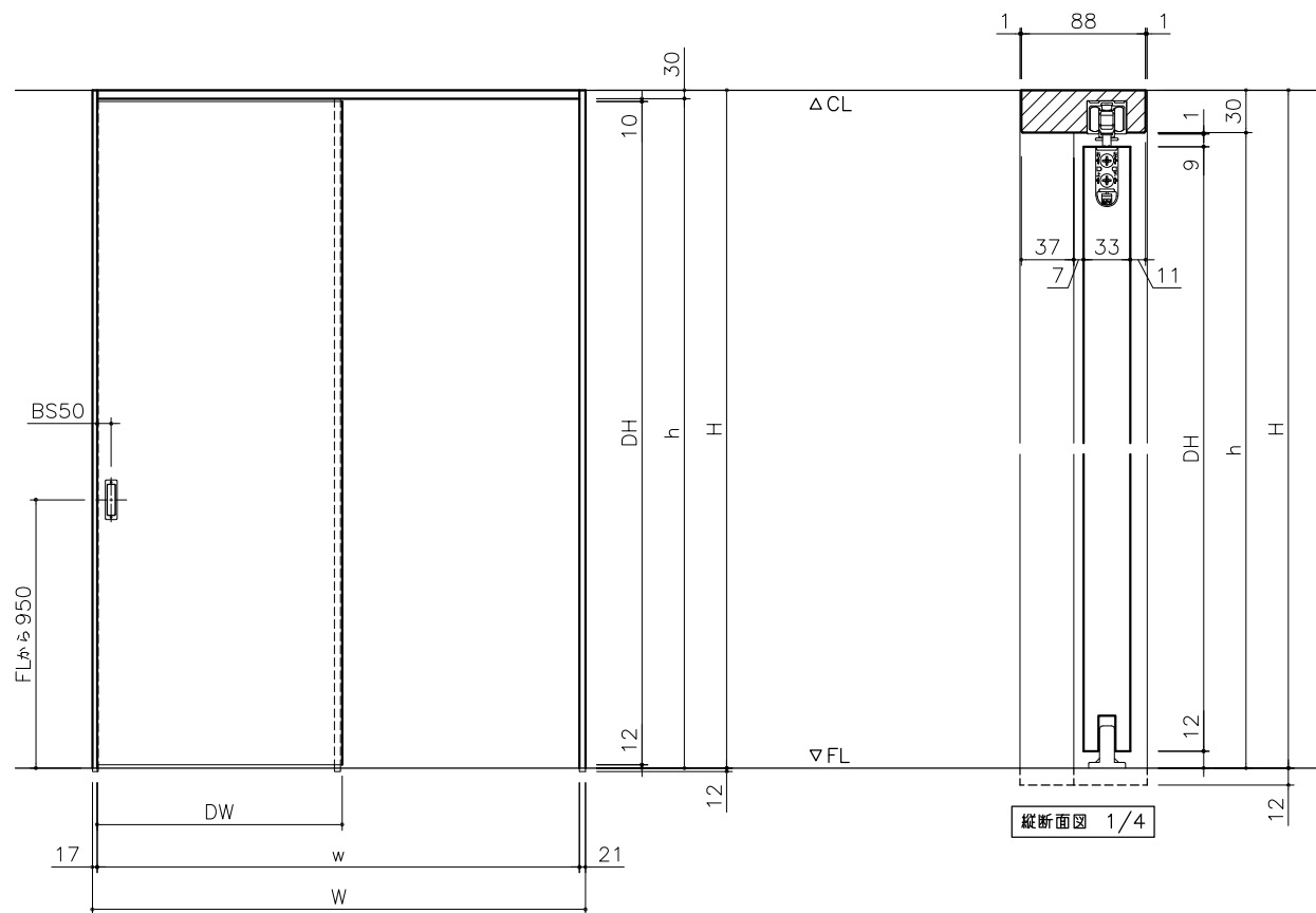
正面図 1/20
