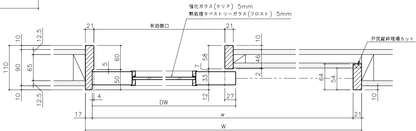
横断面図 1/4
