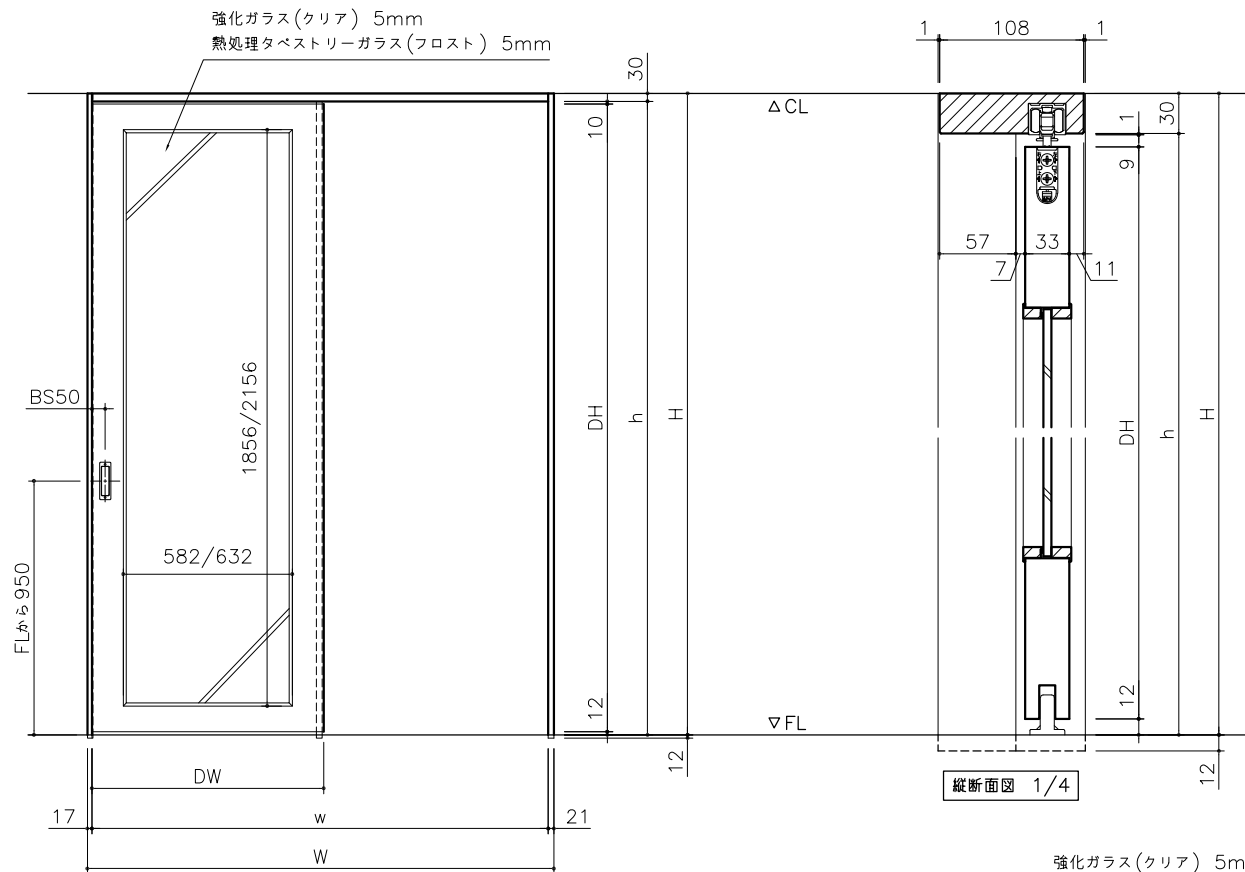
正面図 1/20
