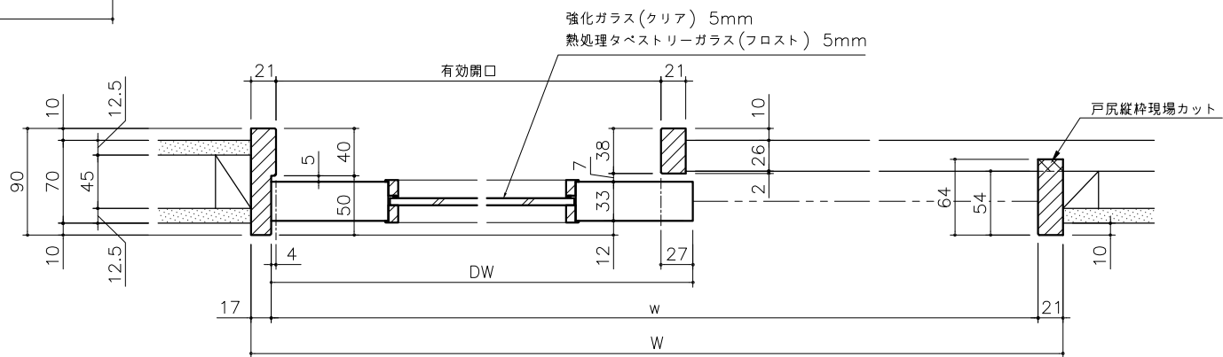
正面図 1/20
