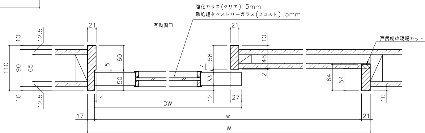
横断面図 1/4
