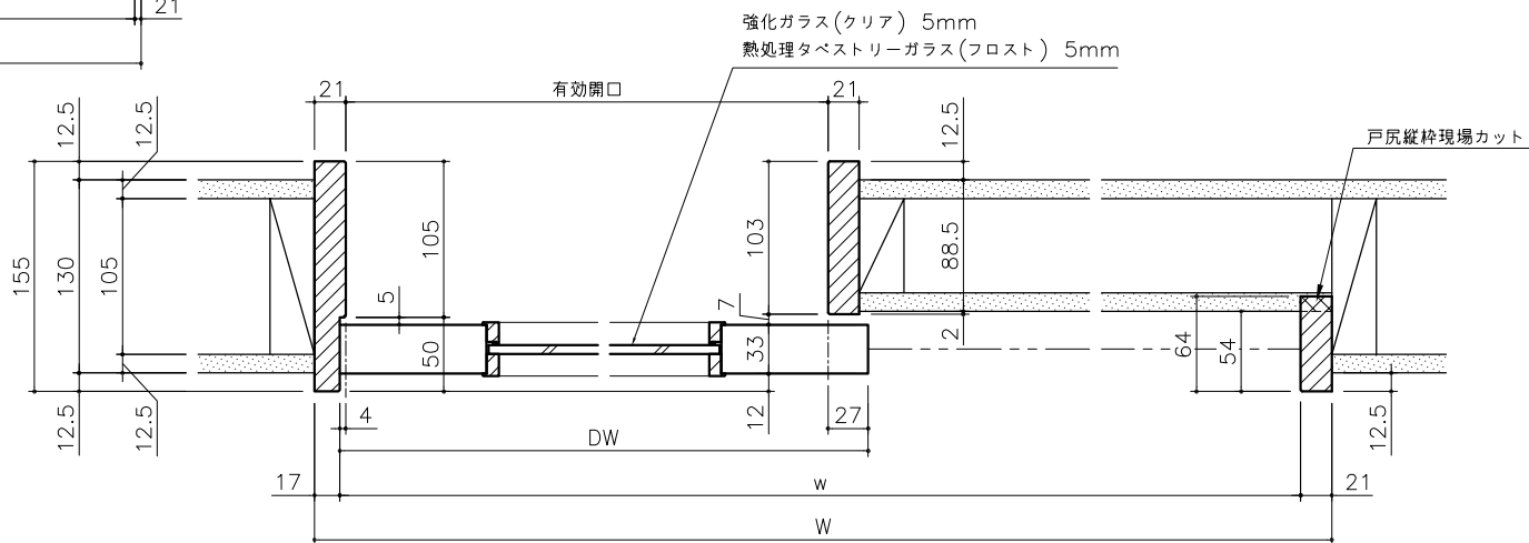
横断面図 1/4
