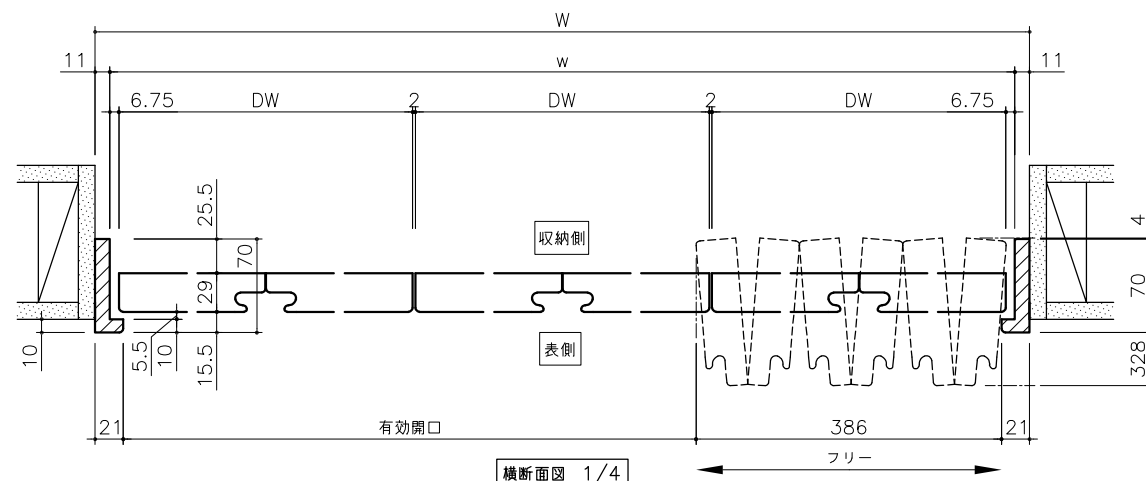
横断面図 1/4
