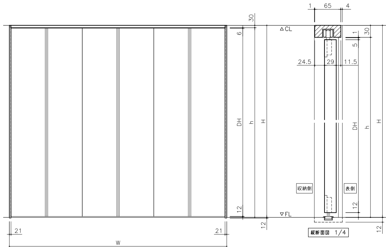
正面図 1/20
