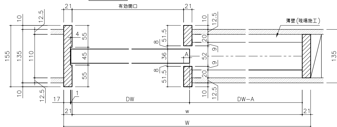
横断面図 1/4
