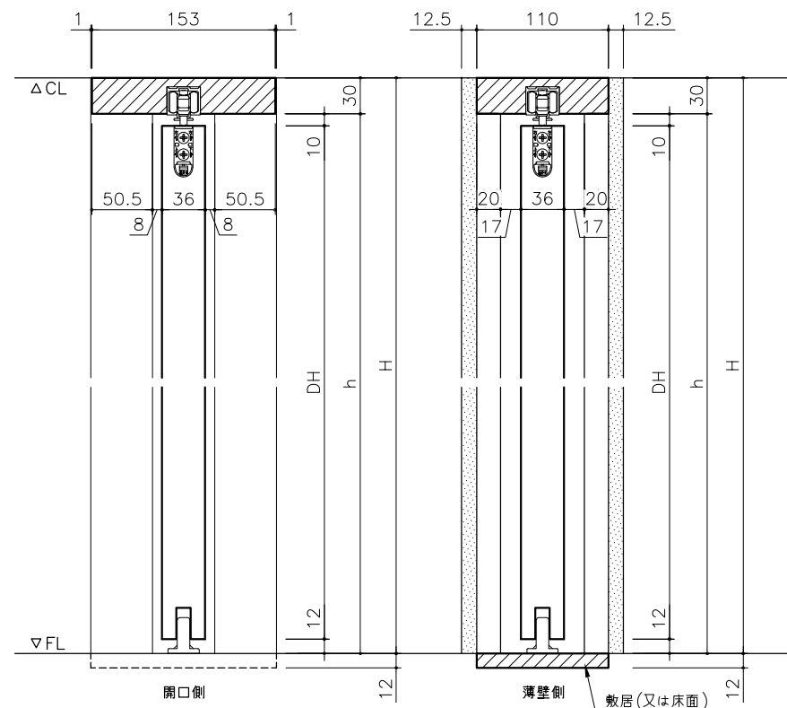
縦断面図 1/4
