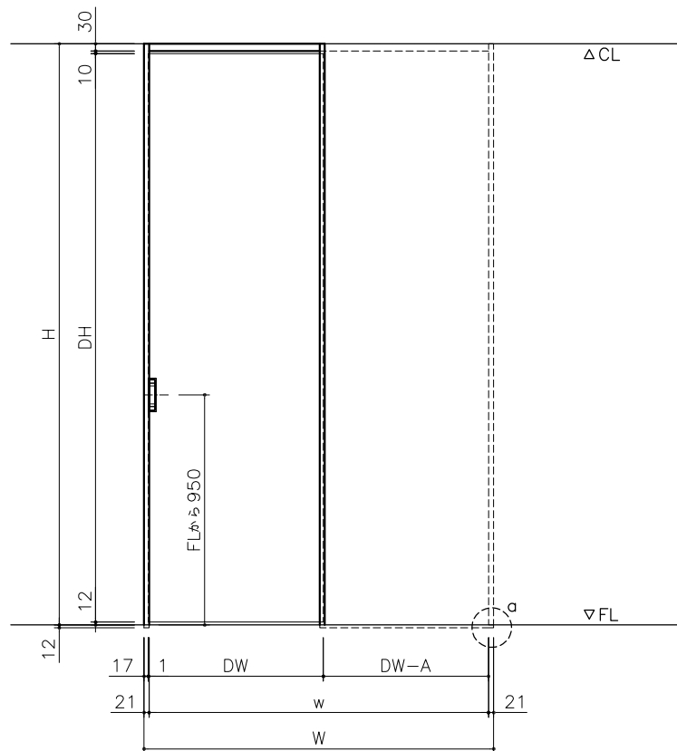
正面図 1/20
