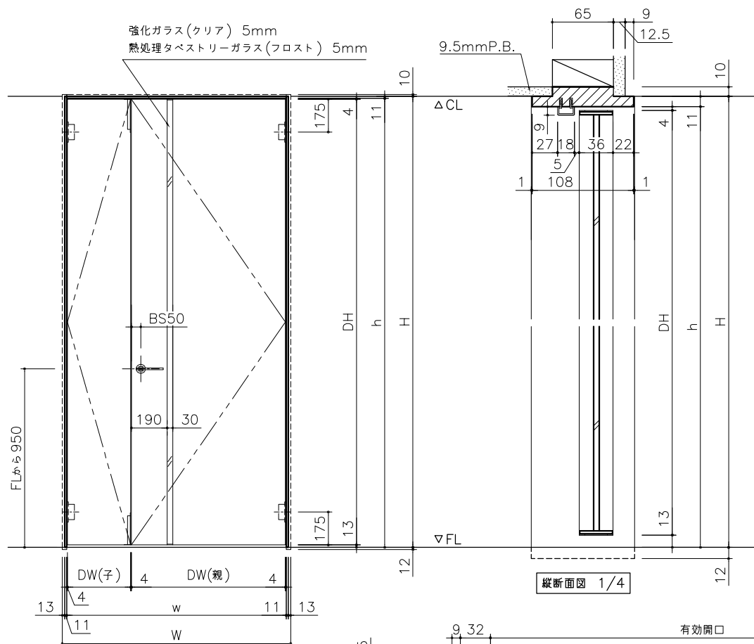
正面図 1/20
