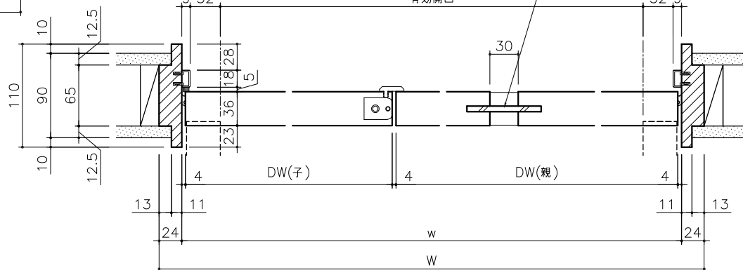
横断面図 1/4
