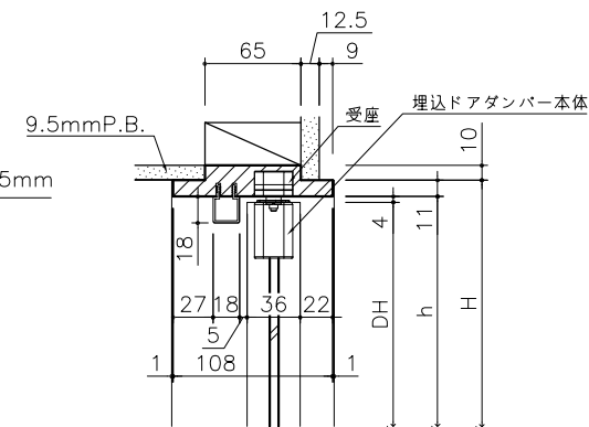
縦断面図 1/4
