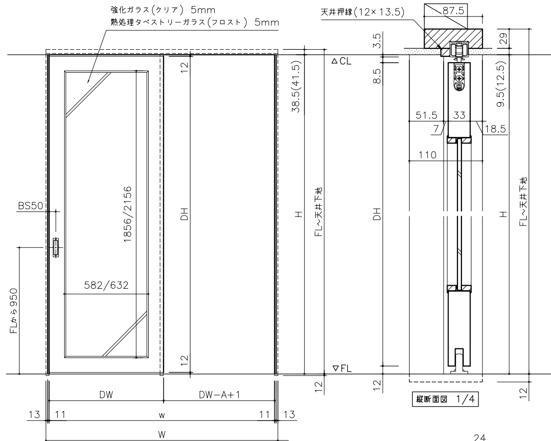
正面図 1/20 * ( )内寸法はP.B.12.5mmの場合を示す。
