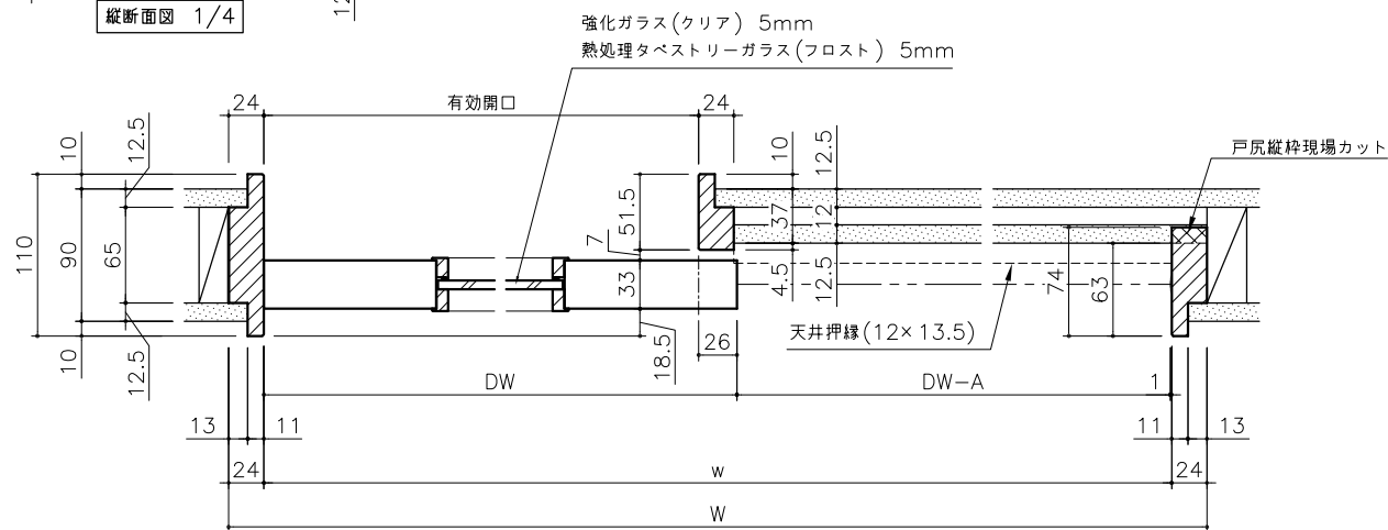
横断面図 1/4
