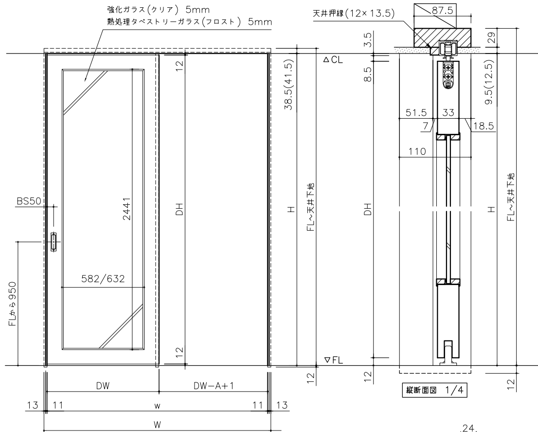
正面図 1/20 * ( )内寸法はP.B.12.5mmの場合を示す。
