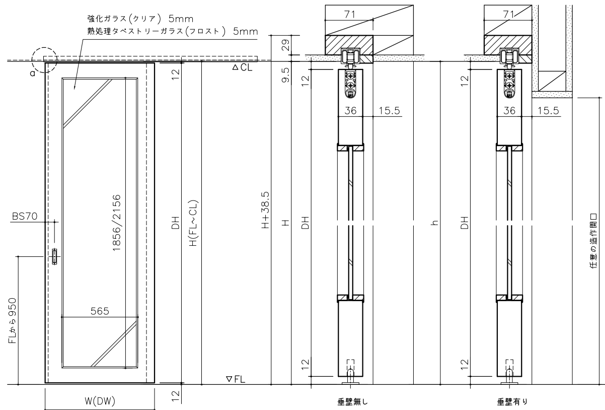
縦断面図 1/4
