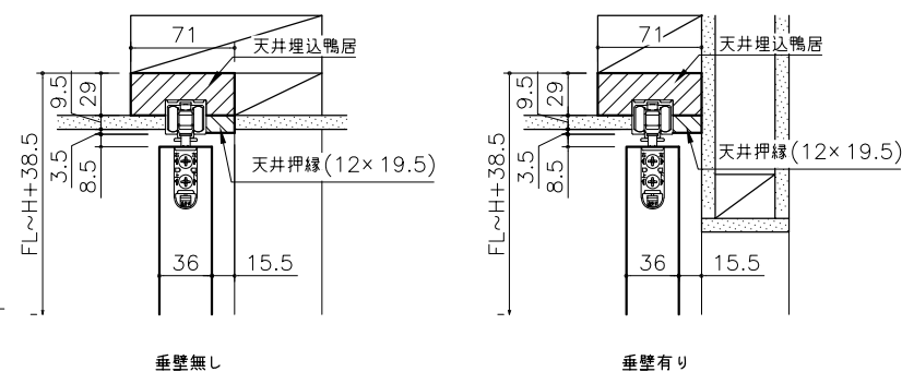
縦断面詳細図 1/4
