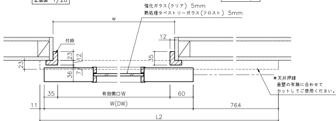
横断面図 1/4
