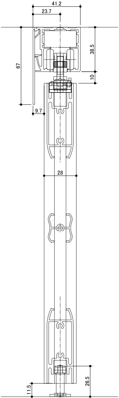
側面 詳細図 S=1:2
