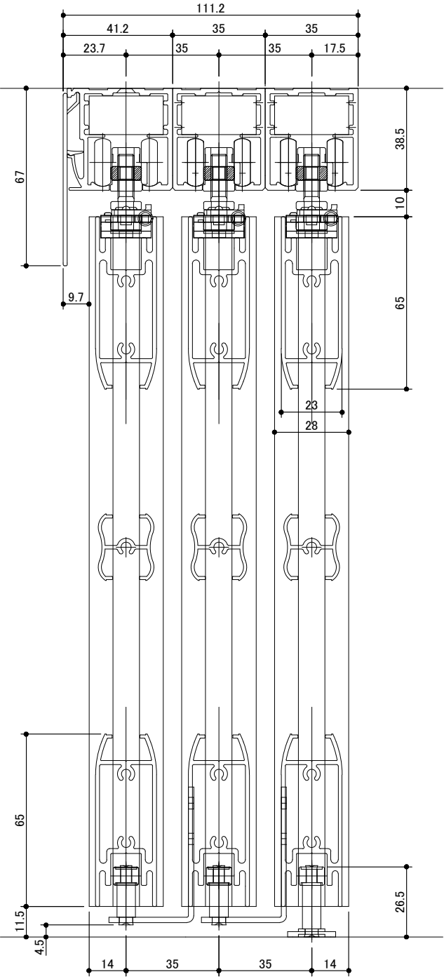
側面 詳細図 S=1:2
