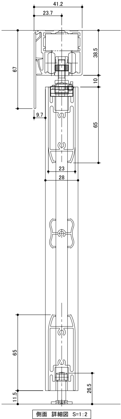
側面 詳細図 S=1:2
