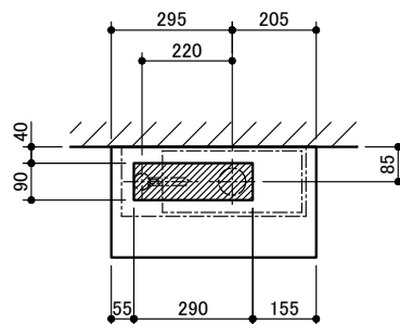
左水栓
