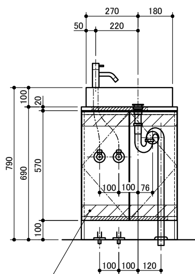
混合水栓
