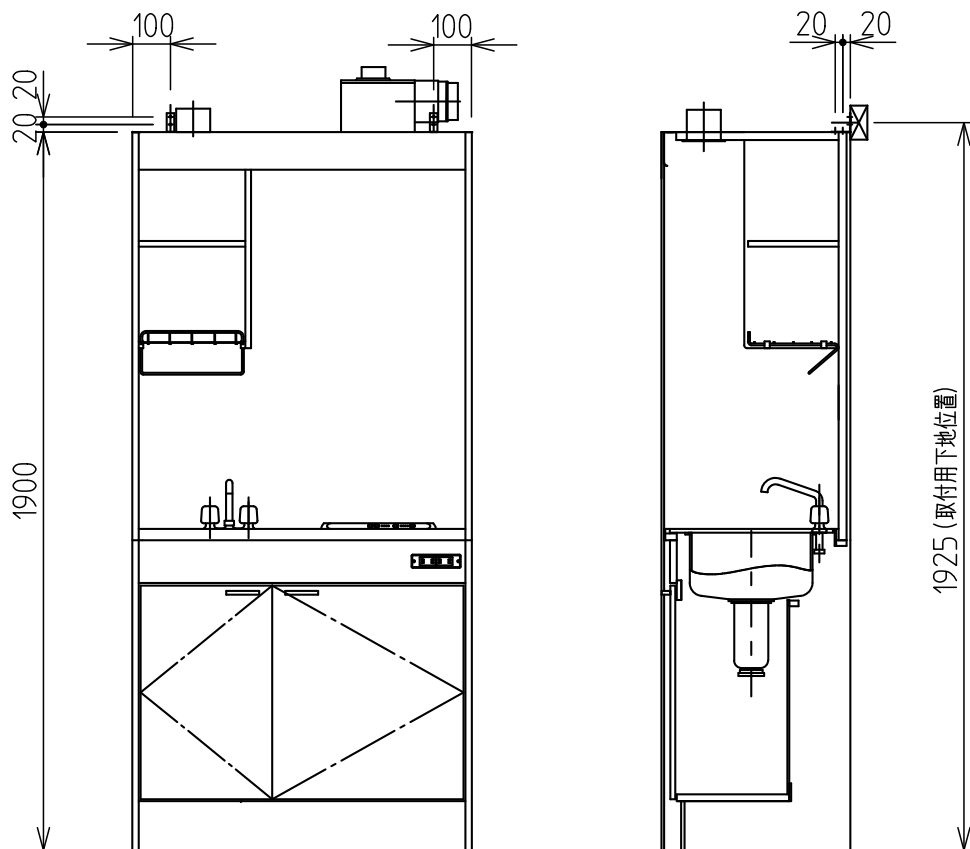
上下ユニット固定位置
