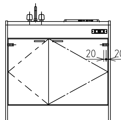
下部ユニット（ハーフタイプ）固定位置
