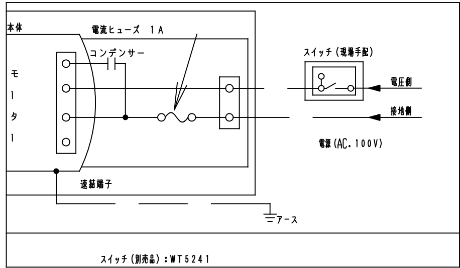
□ 結線図
