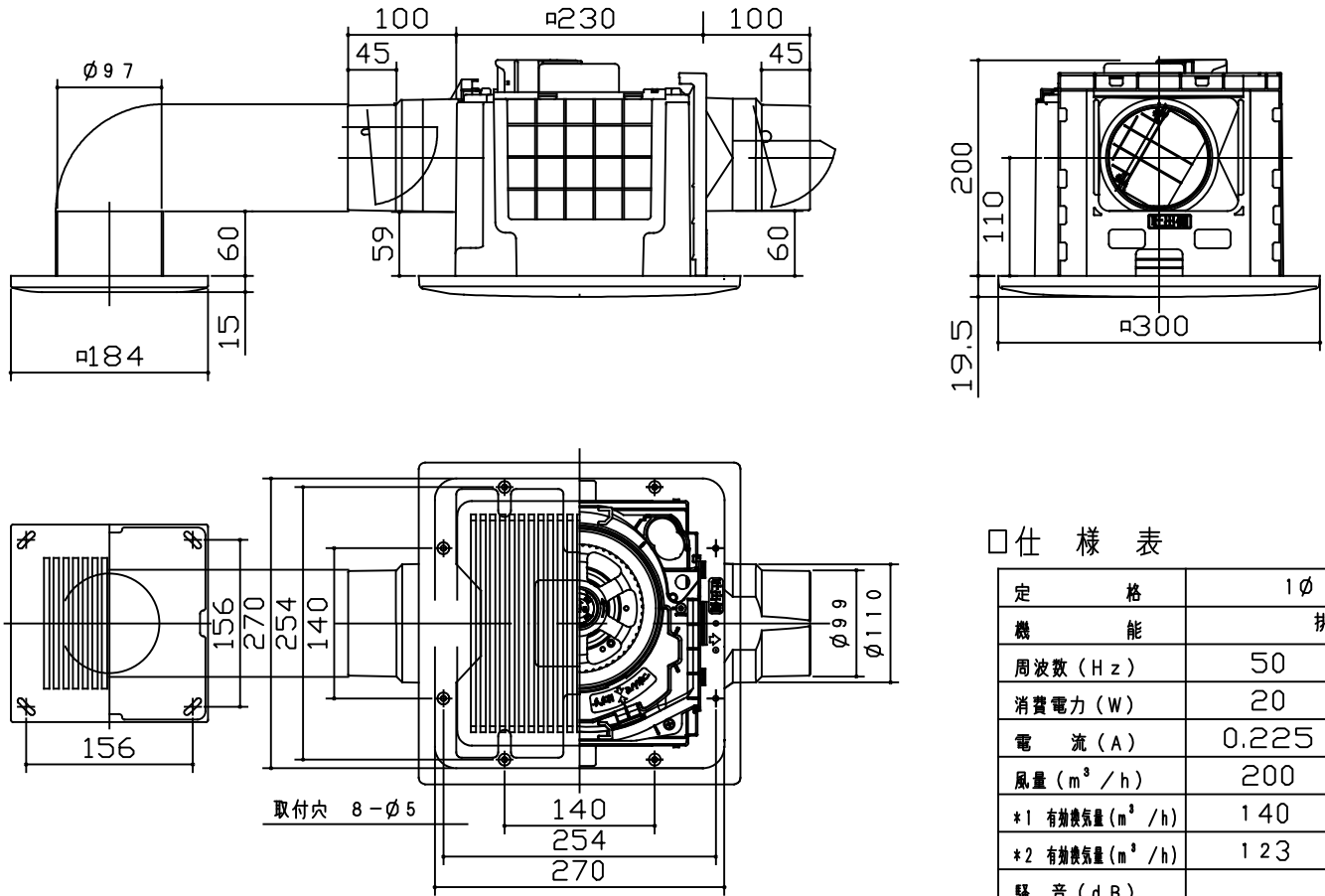
□ 寸法図
