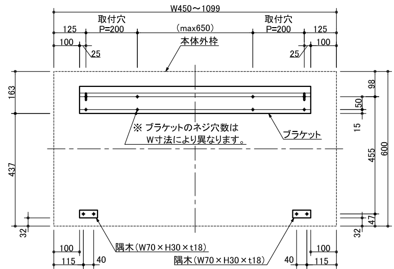
ブラケット・隅木の壁取付位置関係図
