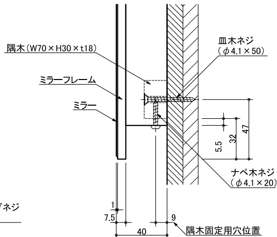
B 詳細図 S=1:3
