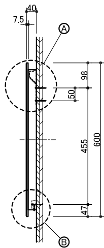
側面図
