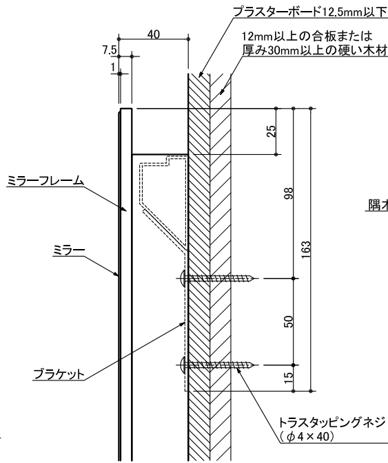
A 詳細図 S=1:3
