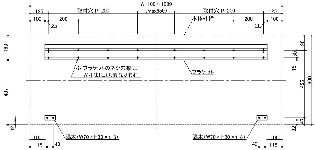
ブラケット・隅木の壁取付位置関係図
