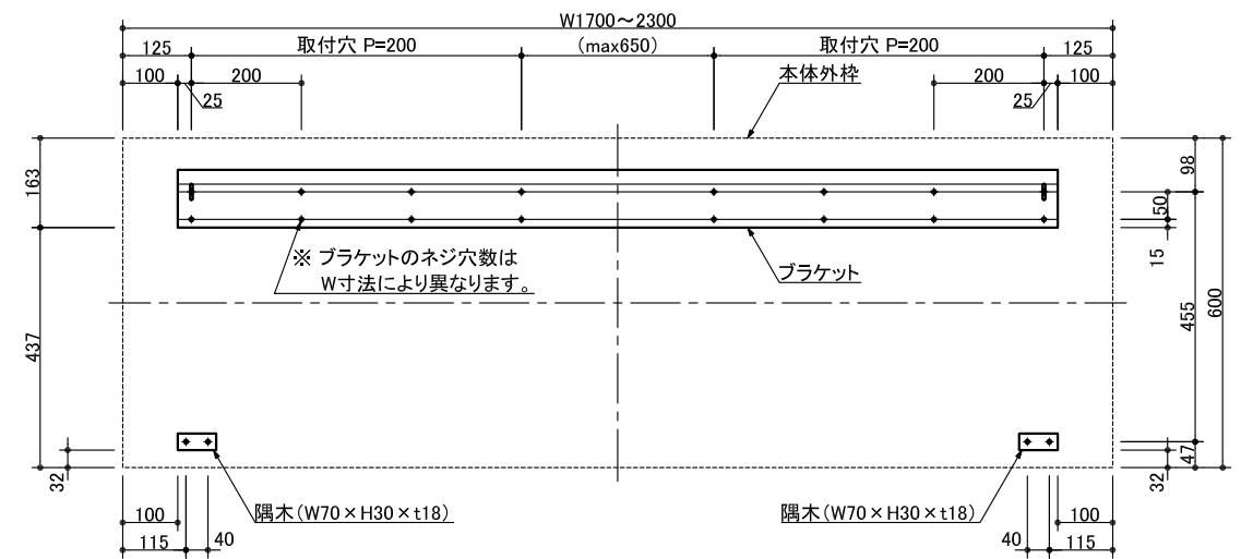
ブラケット・隅木の壁取付位置関係図
