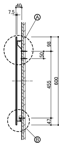
側面図
