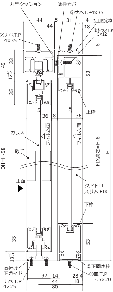
側面図詳細
