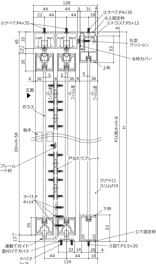
側面図詳細
