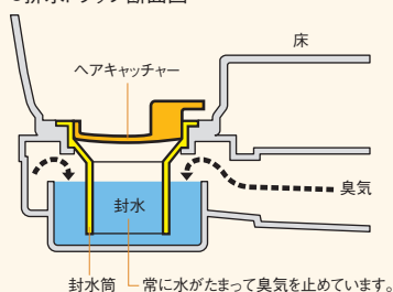
●排水トラップ断面図
