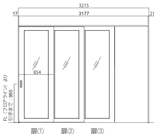
《正面図》
