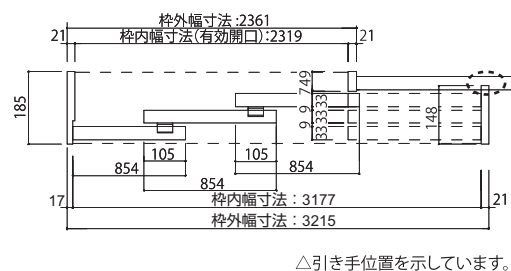
《横断面図》
