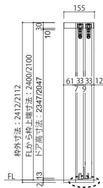
《縦断面図》
