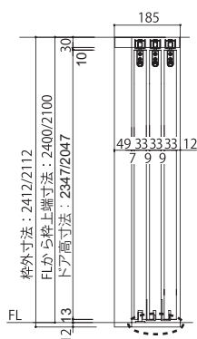
《縦断面図》
