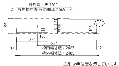
《横断面図》
