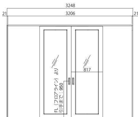
《正面図》
