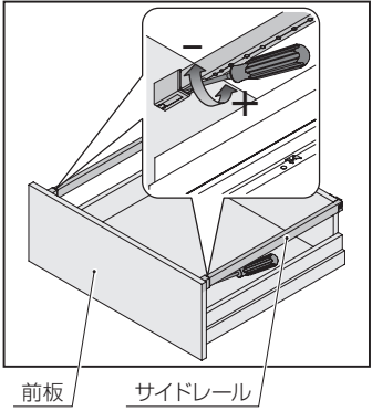
上下調整 ± 2mm
