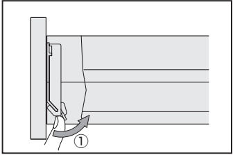
左右調整 ± 1.5mm
